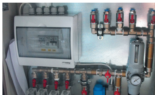
Nowe szafy sterownicze na SUW
